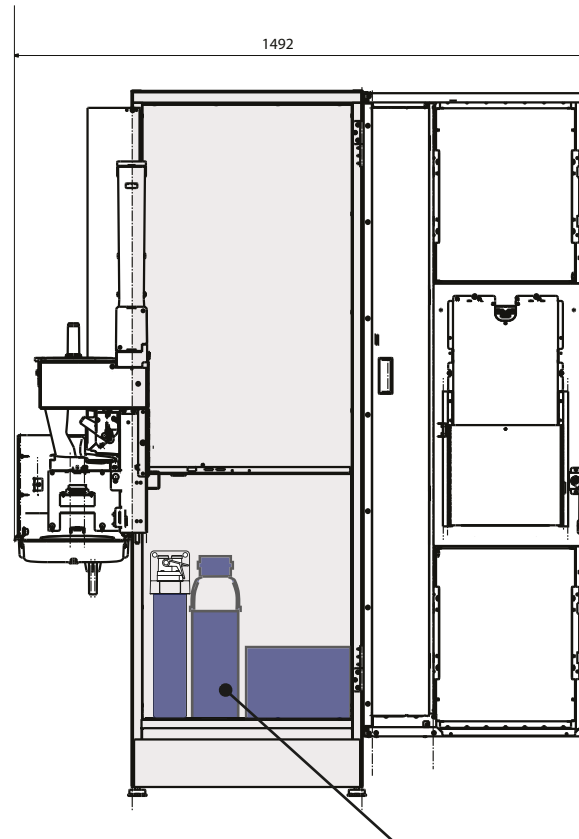
Positie van filters / optionele koud water unit
